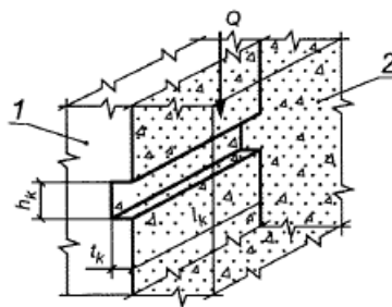
1 - сборный элемент; 2 - монолитный бетон
