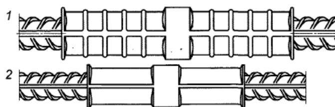
1 - с промежутками; 2 - без промежутков
